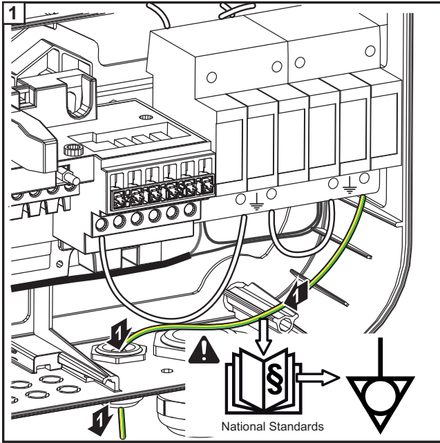
Option DC OVP Typ 2 - M
